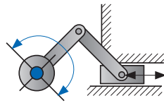
Kurbeltrieb
