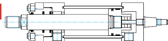
Version mit externen Signalwandler. Für Befestigungen X, A, E, G, L, R. Version with external transducer. For mountings X, A, E, G, H, L, R.
