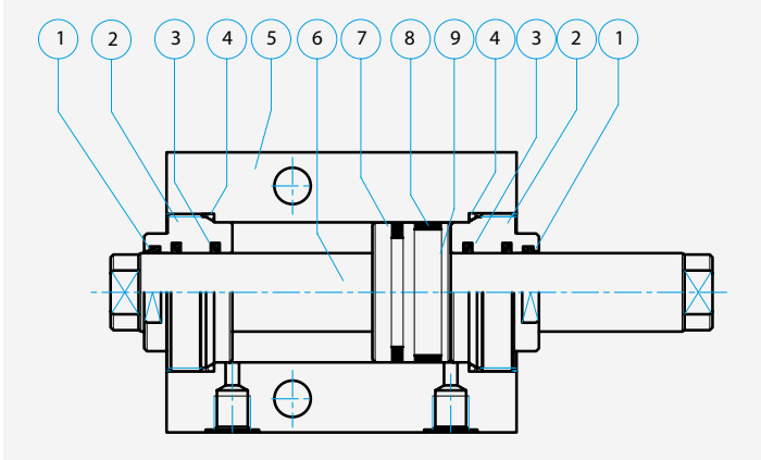
ZYLINDER MIT ZWEIFACHER KOLBENSTANGE
